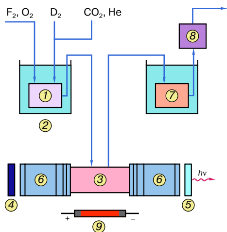
Рис. 6. Схема химического лазера импульсного действия: 1 – смеситель, 2 – холодильник, 3 – реактор, 4 – глухое зеркало, 5 – частично прозрачное зеркало для вывода излучения, 6 – держатели окон и камеры защиты окон от коррозии продуктами реакции, 7 – гаситель пламени, 8 – химический поглотитель, 9 – импульсная лампа – источник иницирующего излучения
